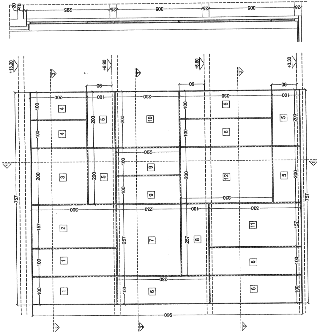
ИЗГЛЕД
