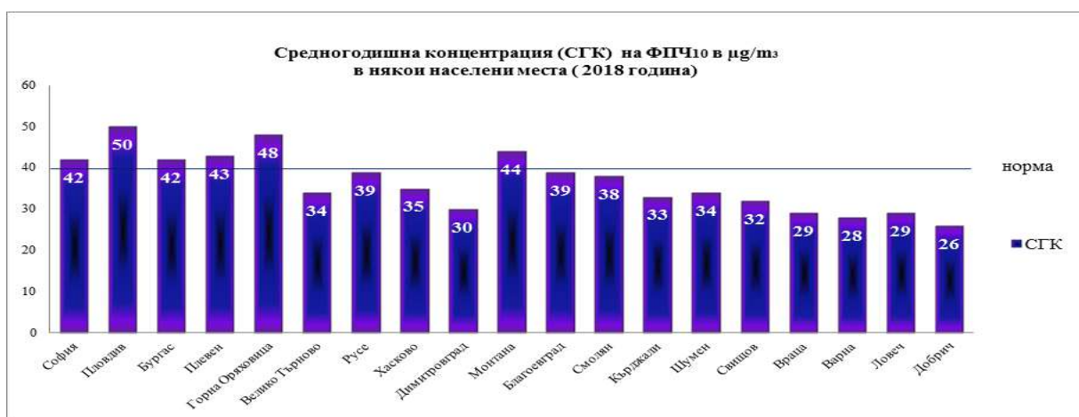
Фигура 59. Средногодишна концентрация на ФПЧ 10
